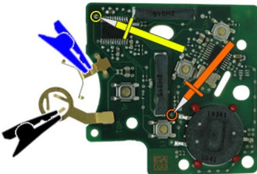
"ZFH-C12 CABLE" (ÜST / TOP)
