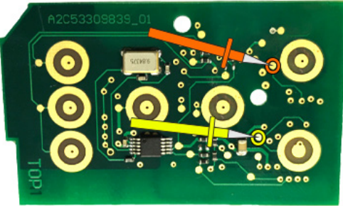
"ZFH-C12 CABLE" (ÜST / TOP)
