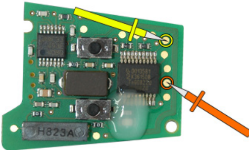
"ZFH-C12 CABLE" (ÜST / TOP)
