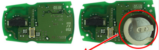
Pil Yatağı Sökülecek / Remove Battery Holder
