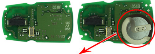
Pil Yatağı Sökülecek / Remove Battery Holder
