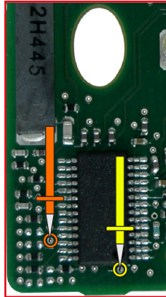
"ZFH-C12 CABLE" (ÜST / TOP)
